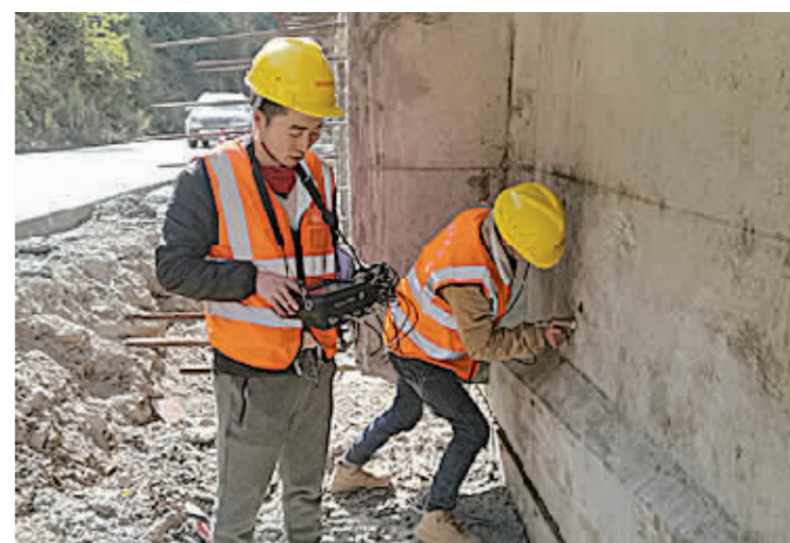
梁板检测现场。
